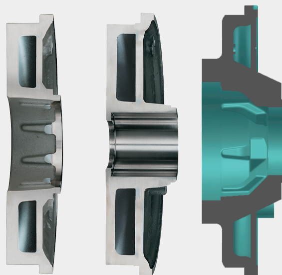
Cámara cónica Cajera cilíndrica FMS/FMI
