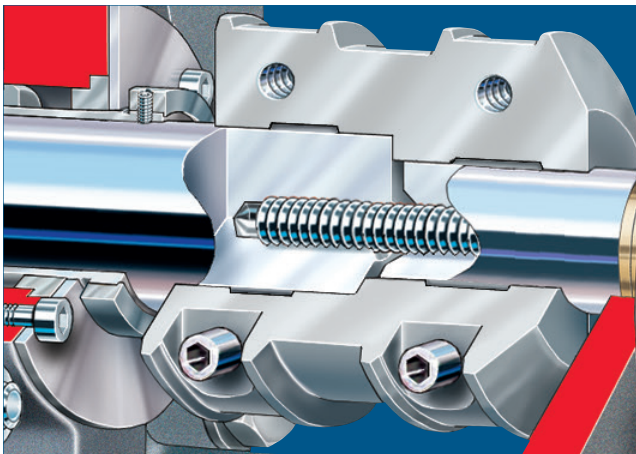
Feinguss-Muffenkupplung (WEB)
