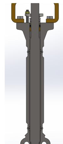
Figure 9 : Chapeau cryogénique
