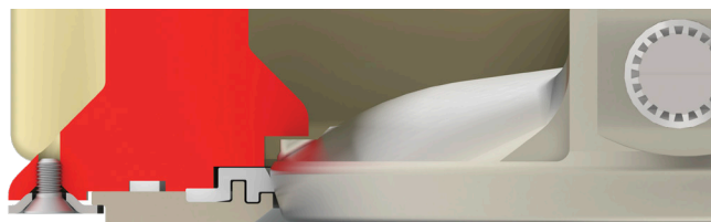
Figure 4 : Disposition du siège souple
