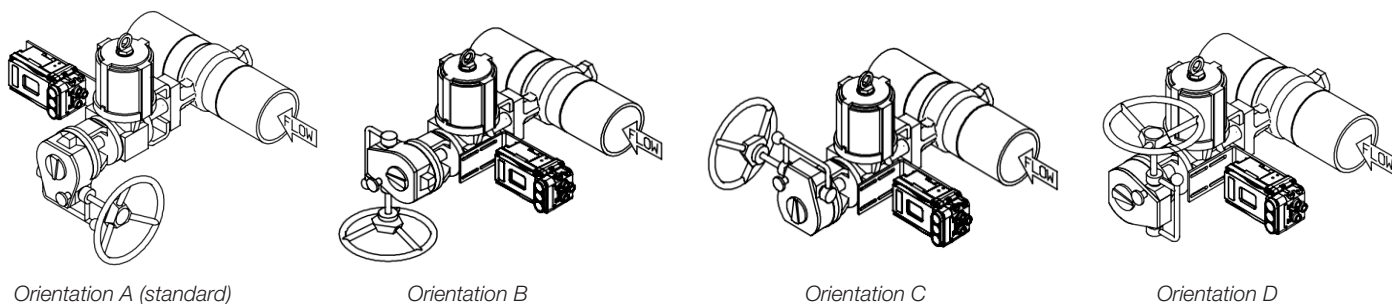
Figure 12 : Orientations du volant
