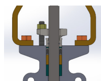
Figure 7 : Chapeau standard
