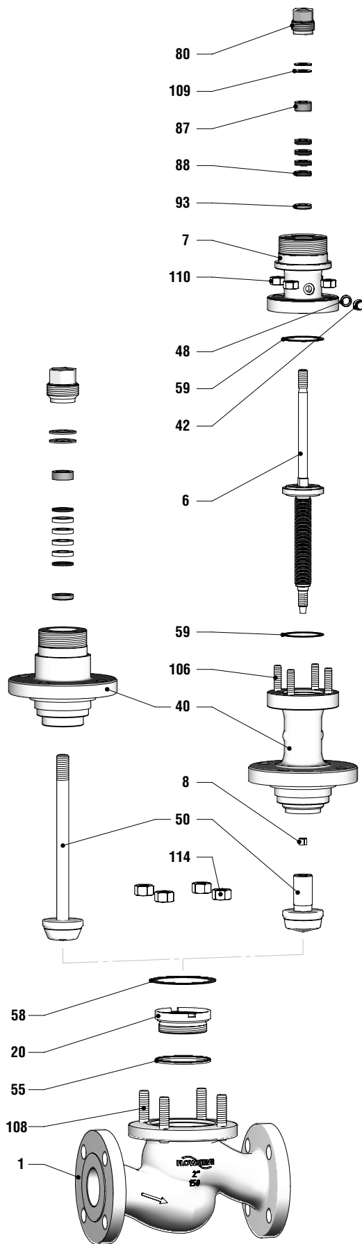
Abbildung 16: Teileübersicht
