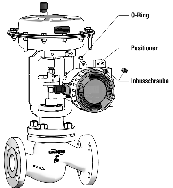
Abbildung 14: Positioner abbauen
