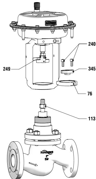
Abbildung 15: Antrieb abbauen
