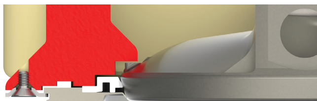
Figura 6: Disposición de asiento doble a prueba de incendio
