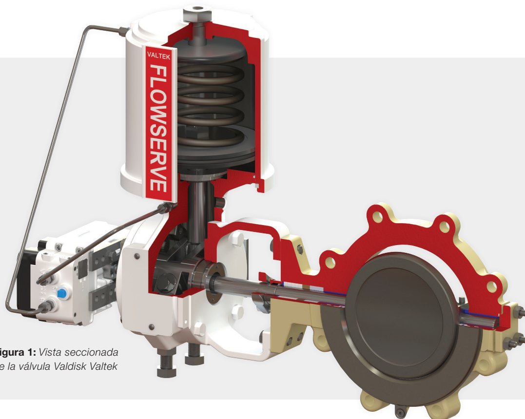
Figura 2: Vista lateral de la válvula Valdisk Valtek que muestra el disco de mariposa de doble excentricidad
